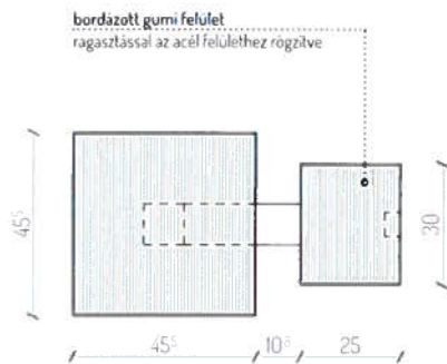
felülnézet ml:20
